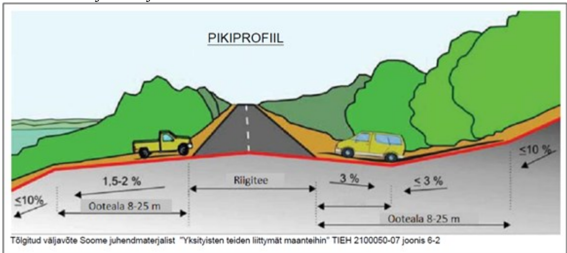
Joonis 2. Ristumiskoha pikikalpede kujundamine
